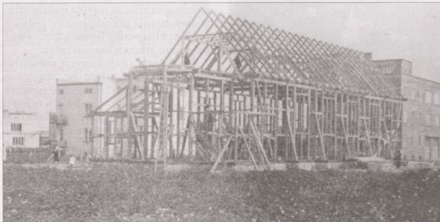
Konstrukcja drewnianego kościółka św. Józefa. Zdjęcie datowane na 8 sierpnia 1943 roku.
